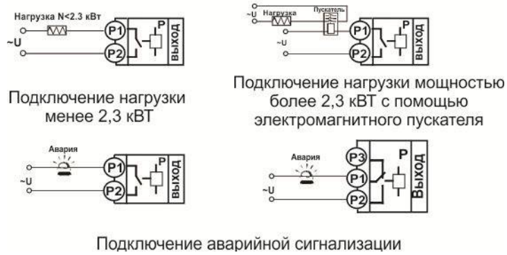
Рисунок 6. Схемы подключения релейных выходов.
